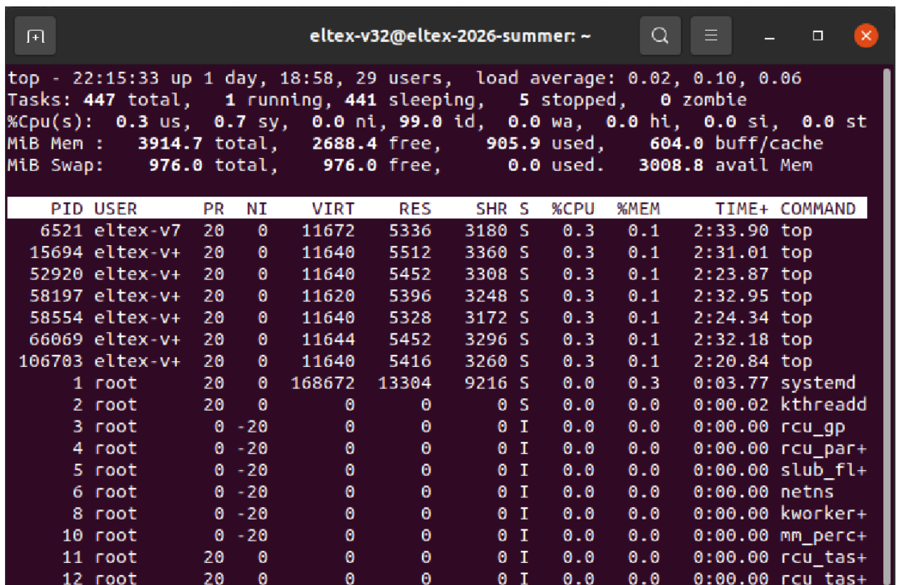
Рис.13. Окно, в котором работает top
