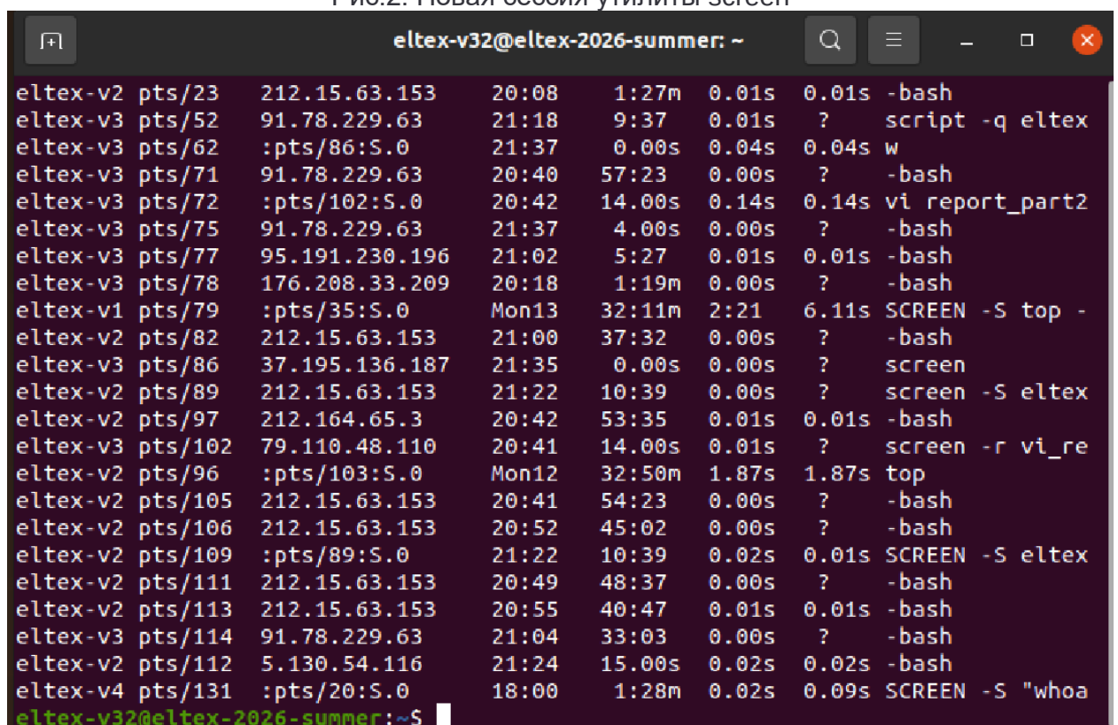
Рис.3. Результат выполнения команды w
